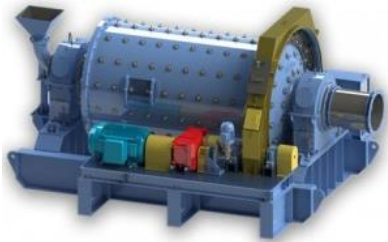
Molinos
